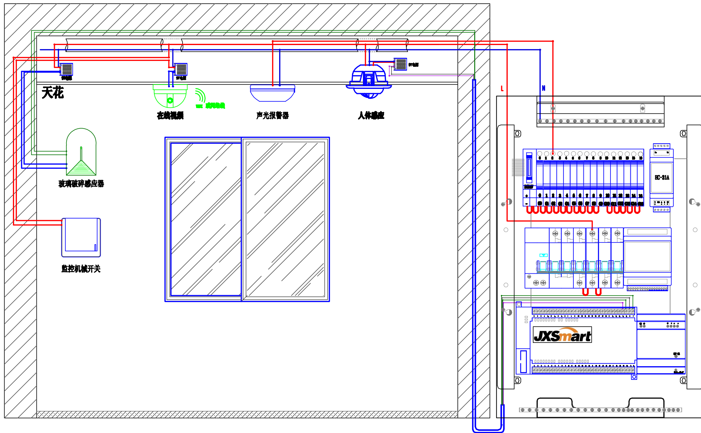
室内安防监控接线方案图
