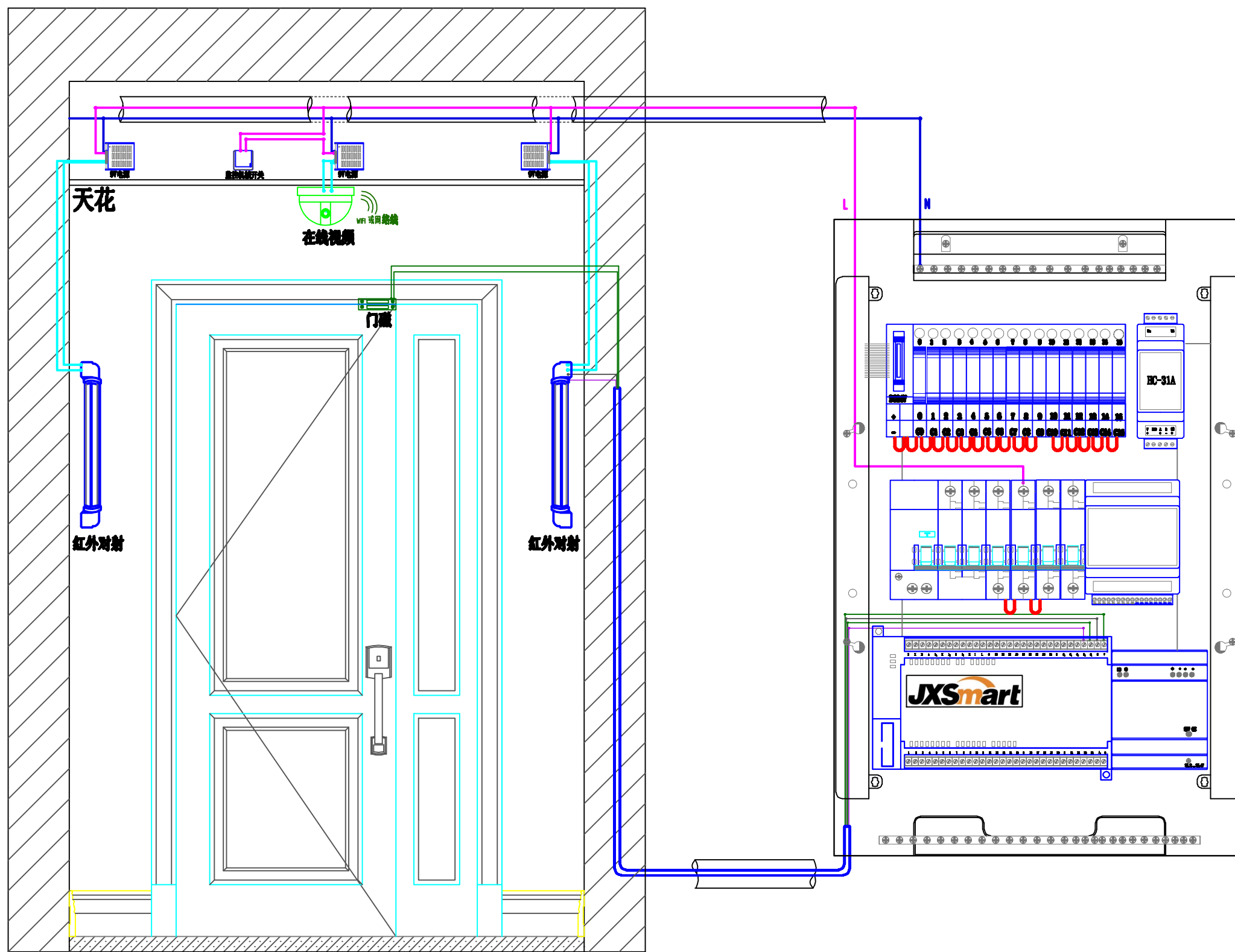
门口安防监控接线方案图
